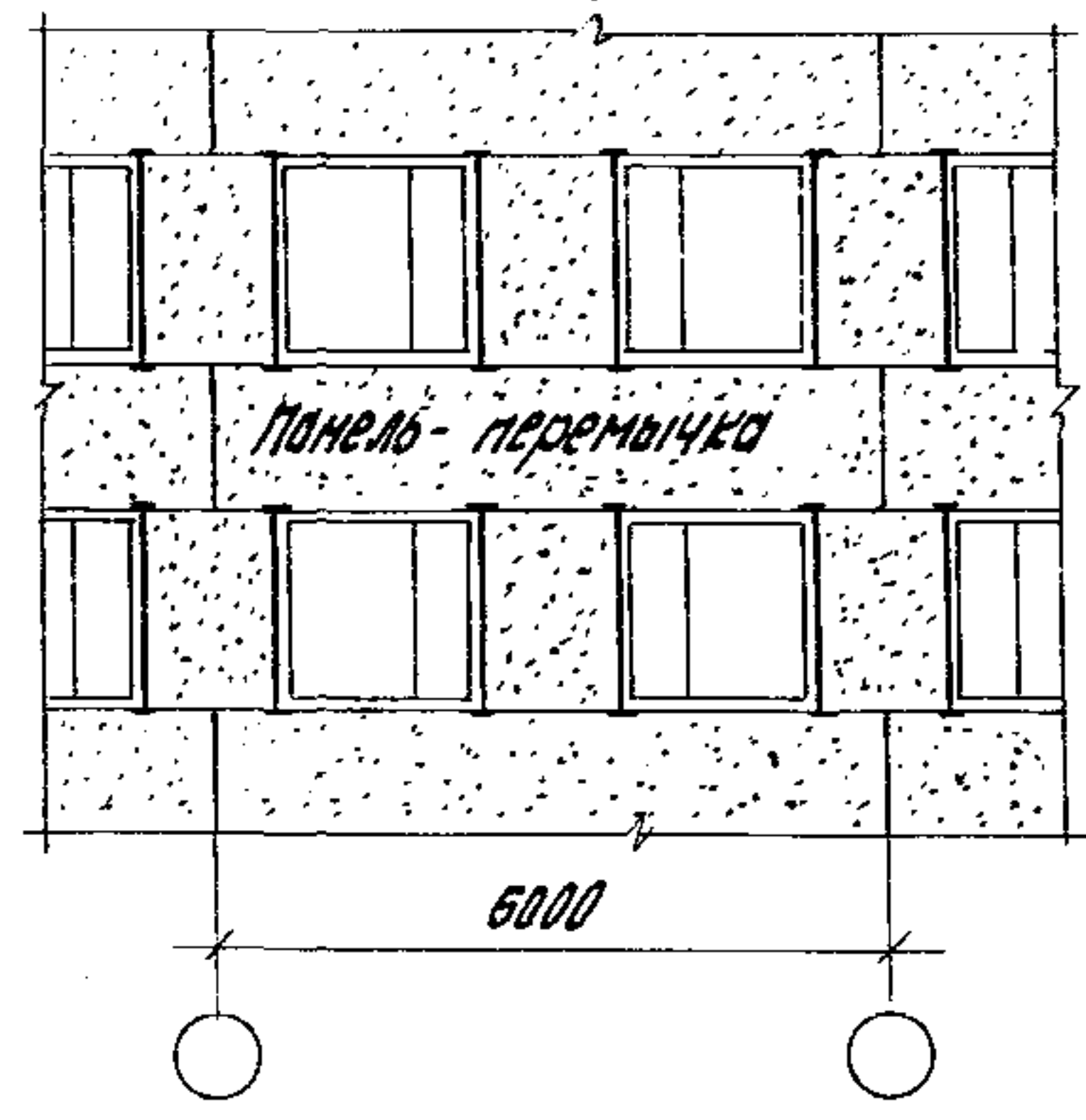
Схема 4. Отдельные проемы шириной 1,8 м Высота окна равна высоте одного простенка ( n \leq 2,4 м)
