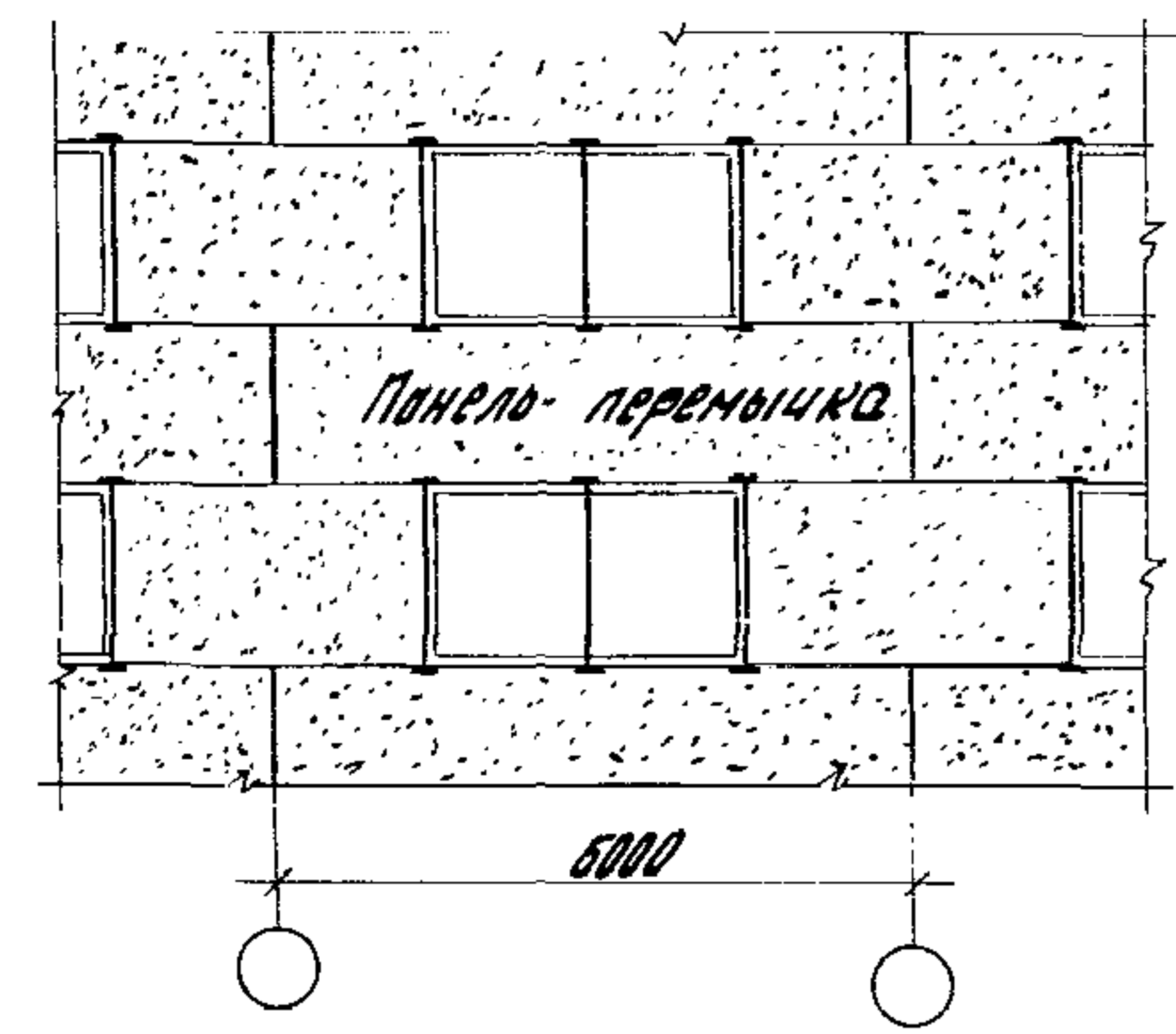
Схема 3. Отдельные проемы шириной 3,0 м. Переплеты с шагом импостов 1,5 м
