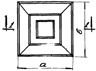
ПЛАН ФУНДАМЕНТА
